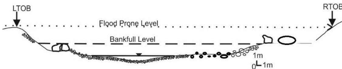
चित्र ५.६ बागमती खोलाको उत्खनन क्षेत्रमा पर्ने भागको cross-section. (Source: Research paper on Bagmati River by Pramila Shrestha, सिचाई विभाग.)
