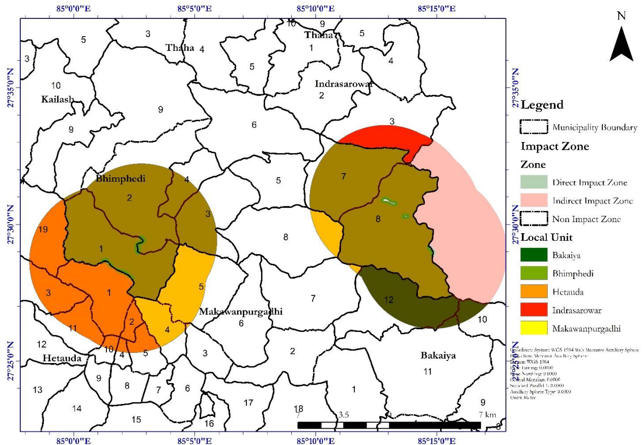
चित्र २.३०: प्रस्तावित आयोजना क्षेत्रको ढुङ्गा, गिट्टी तथा बालुवा उत्खनन/सङ्कलन स्थलको प्रभाव क्षेत्रको नक्सा
