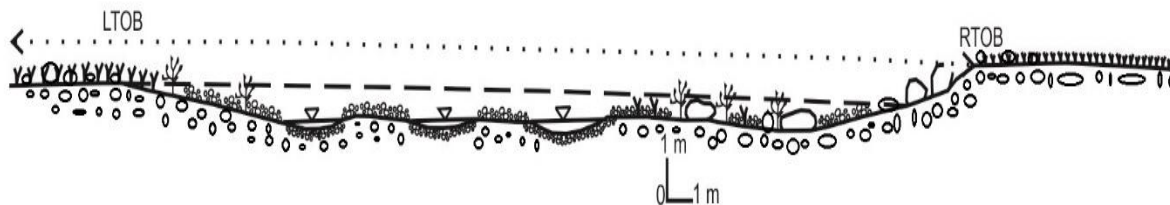
चित्र ५.६: राप्ती खोलाको उत्खनन क्षेत्रमा पर्ने भागको cross-section.
